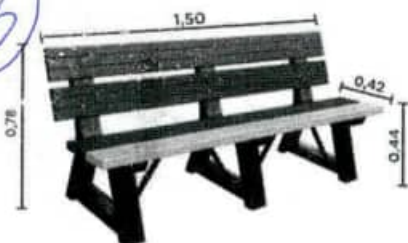
Medidas em metros Banco de Urban Colorido 1,50m
