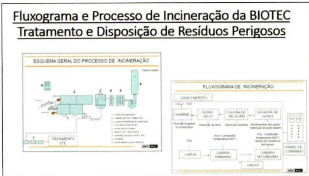
Foto 05 – Fluxograma/Processo de Incineração dos RSS – BIOTEC
