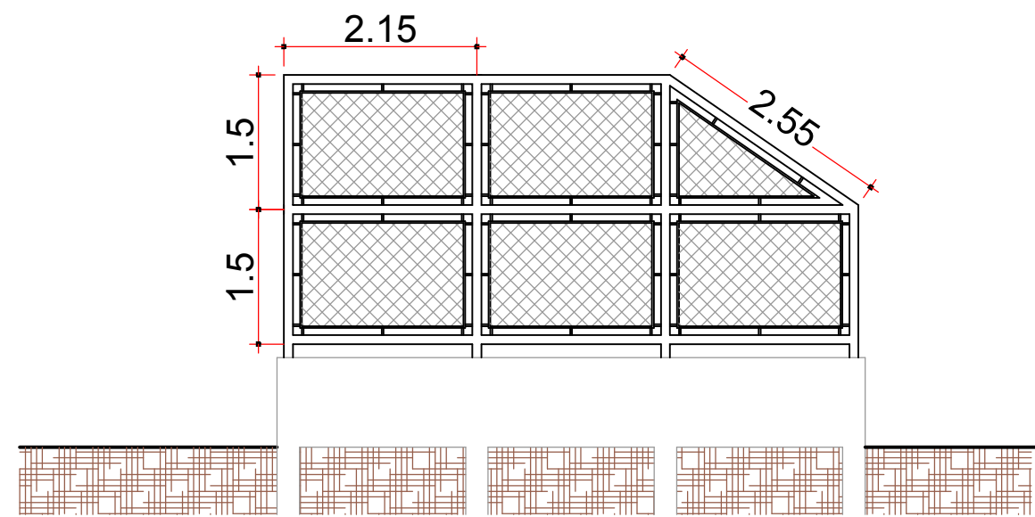
DETALHE ALAMBRADO-LATERAL SEM ESCALA
