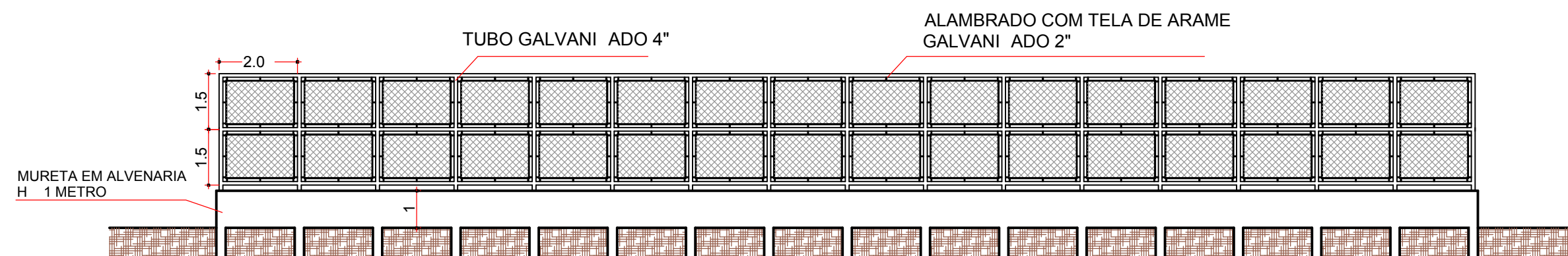
DETALHE ALAMBRADO-LATERAL SEM ESCALA
