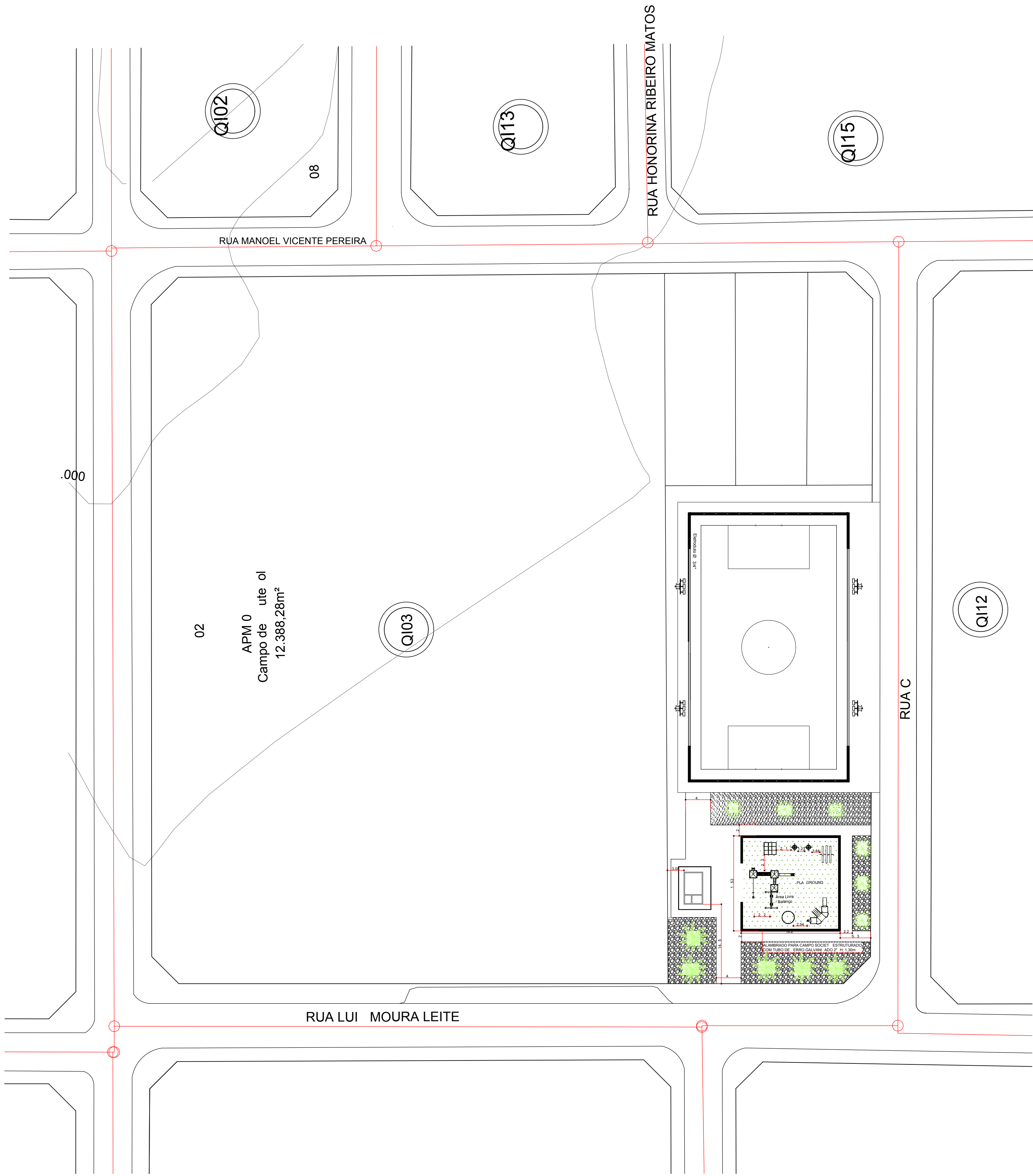
PLANTA DE SITUAÇÃO E LOCAÇÃO ESCALA 1:350
