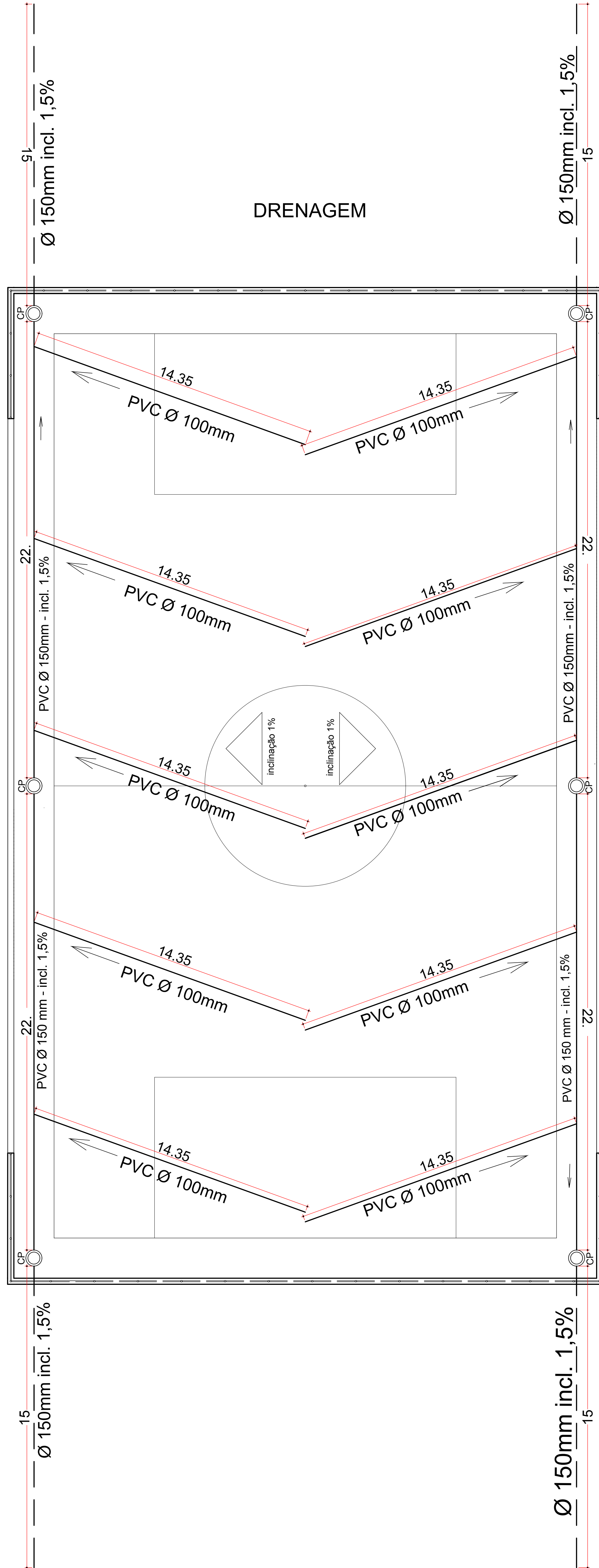
PLANTA BAI A - DRENAGEM ESCALA 1:150
