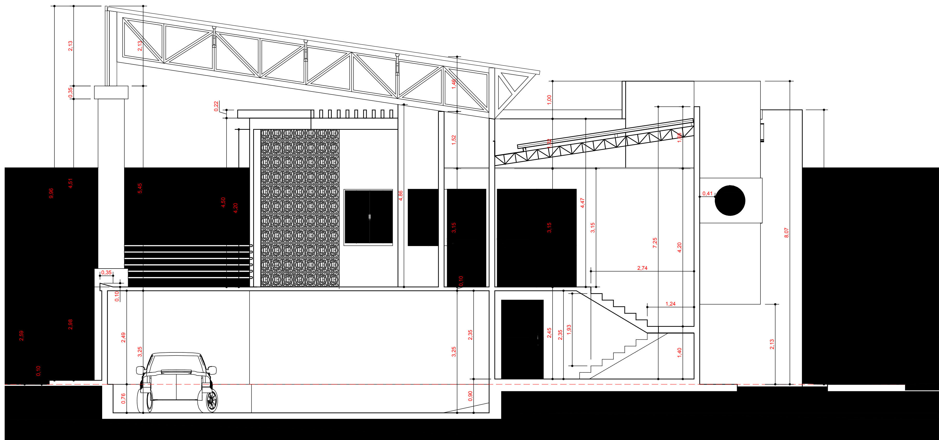
corte C.C
