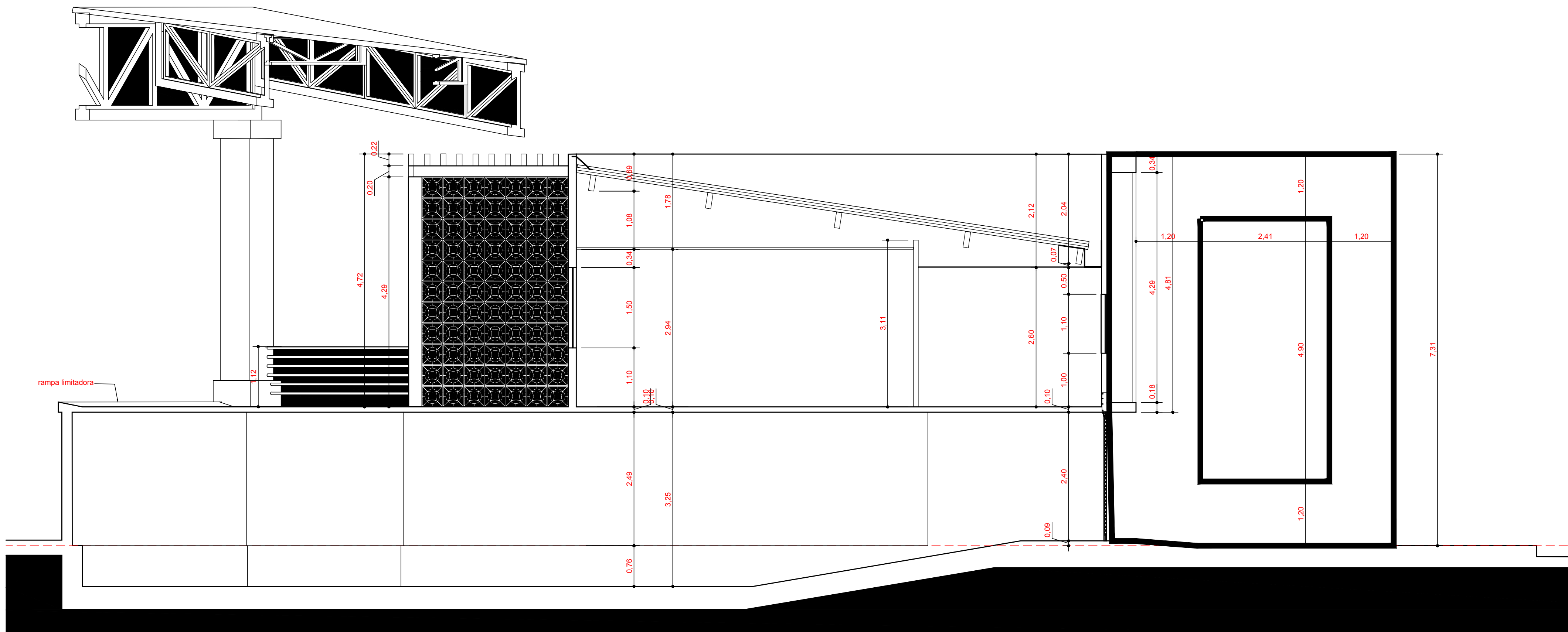
corte A.A
