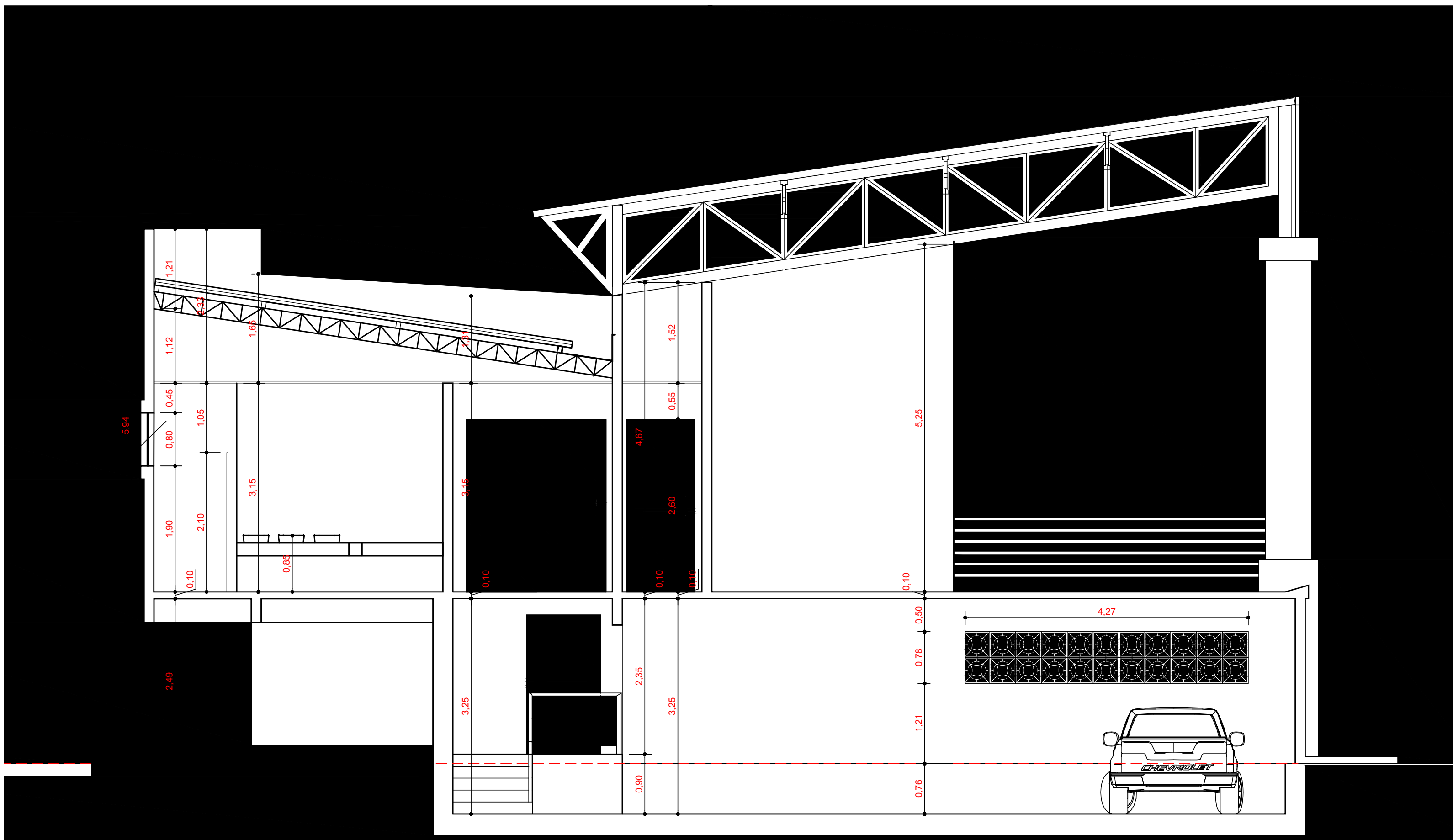
corte B.B
