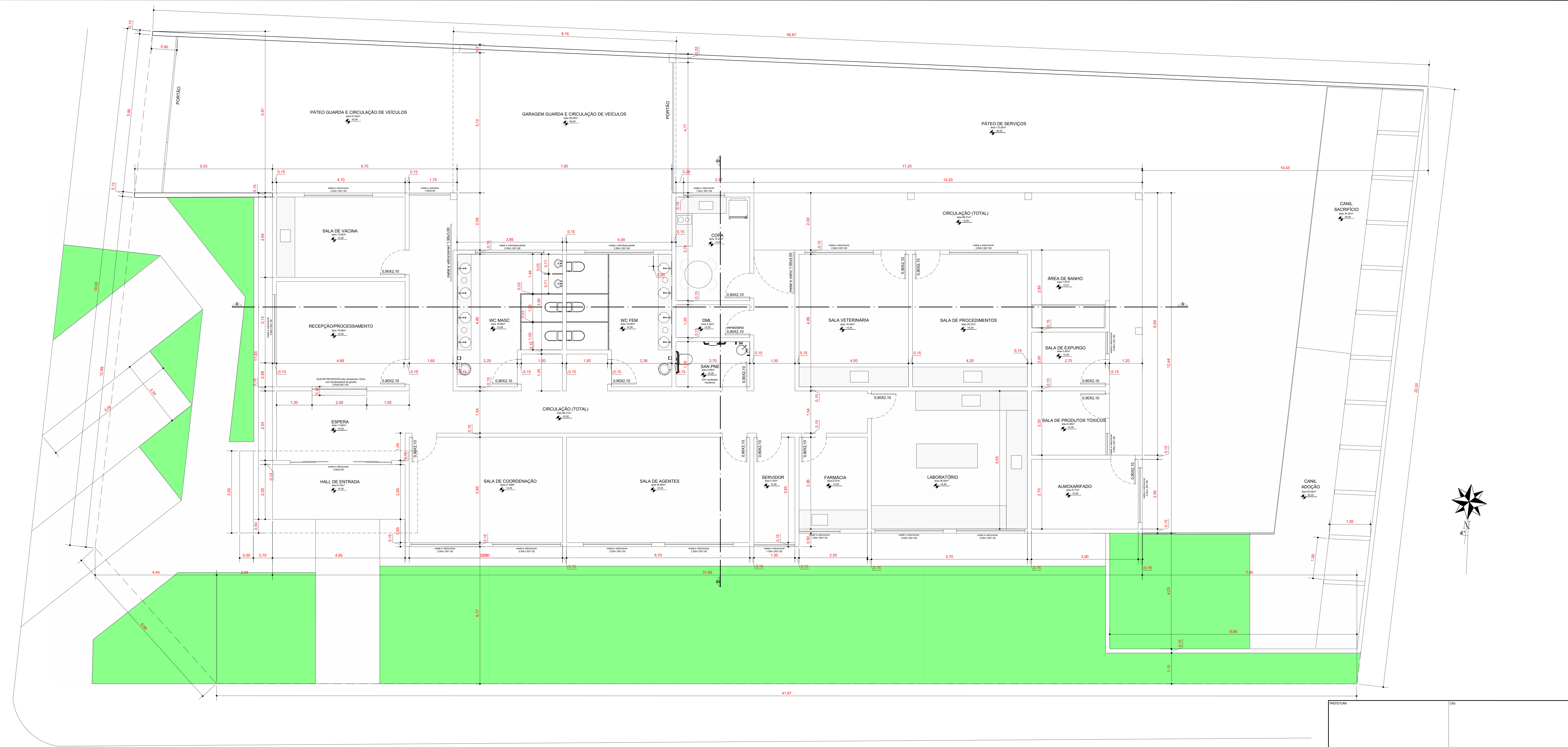
planta baixa
