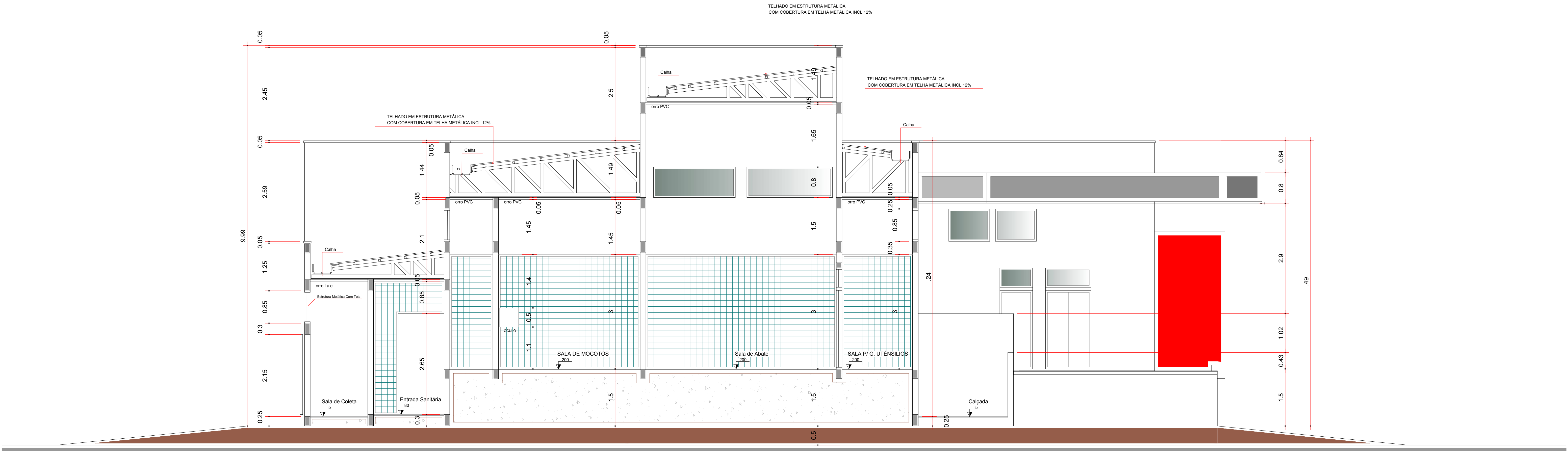
CORTE AA
