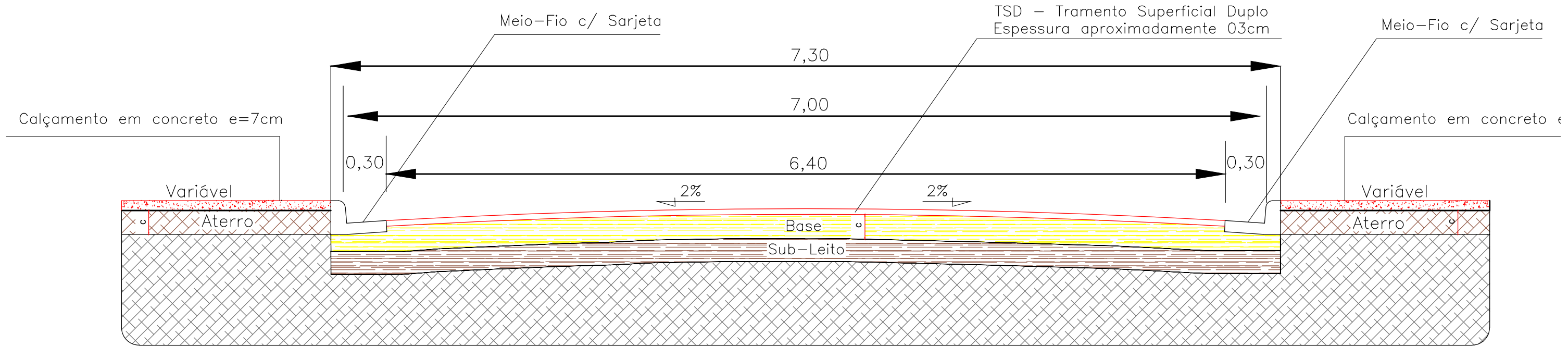
PERFIL TRANS ERSAL - PISTA
