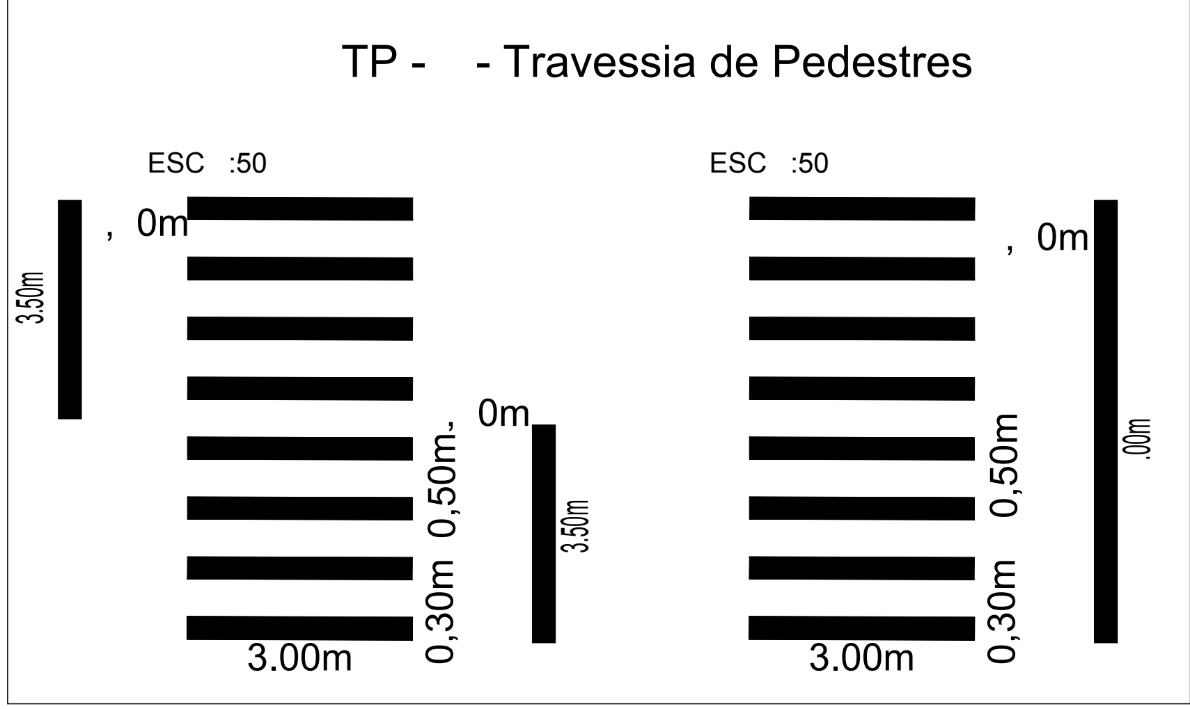
DETALHES AIXA DE PEDESTRE
