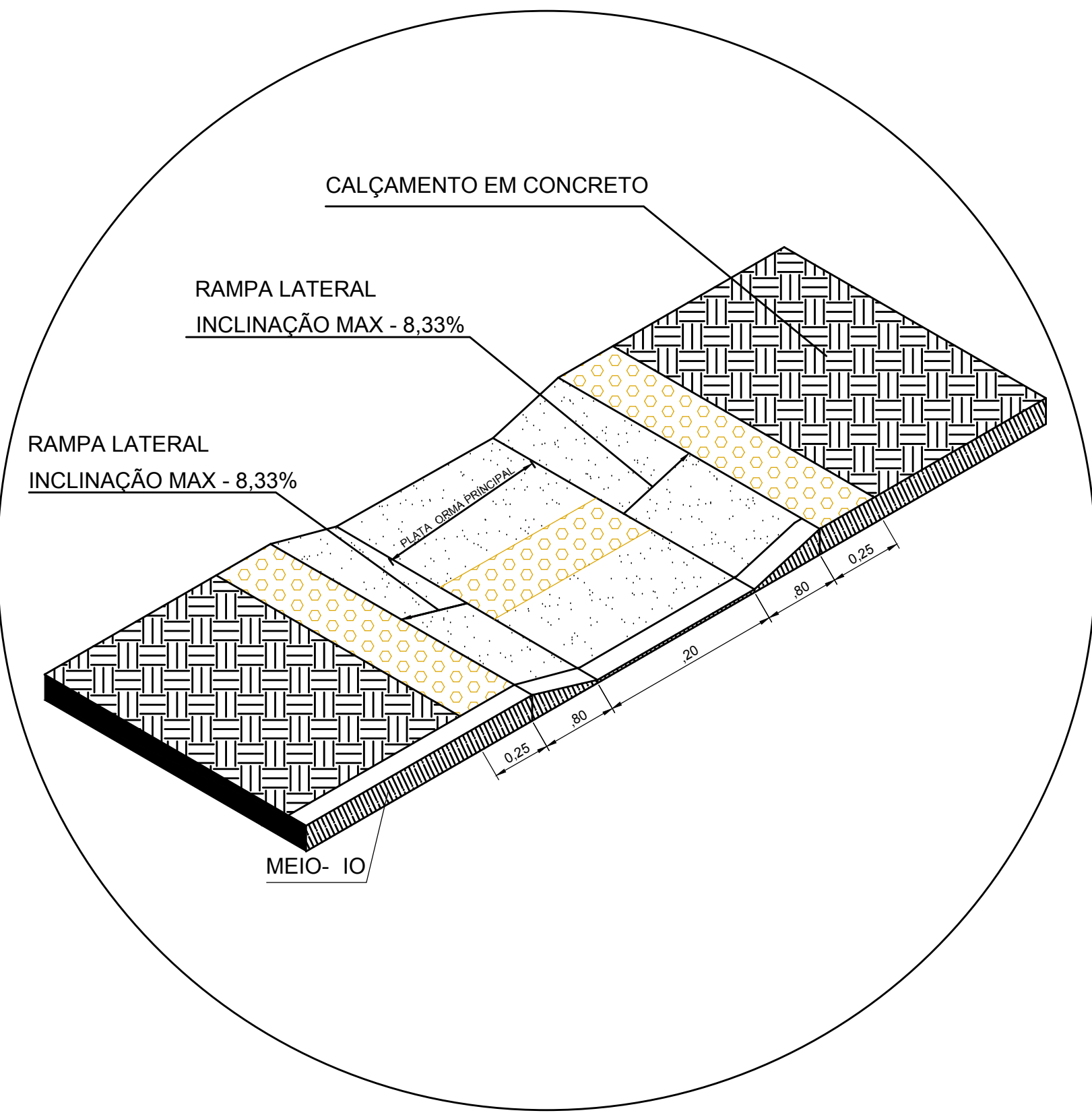
DETALHE DE CALÇADAS COM RAMPA DE ACESSIBILIDADE
