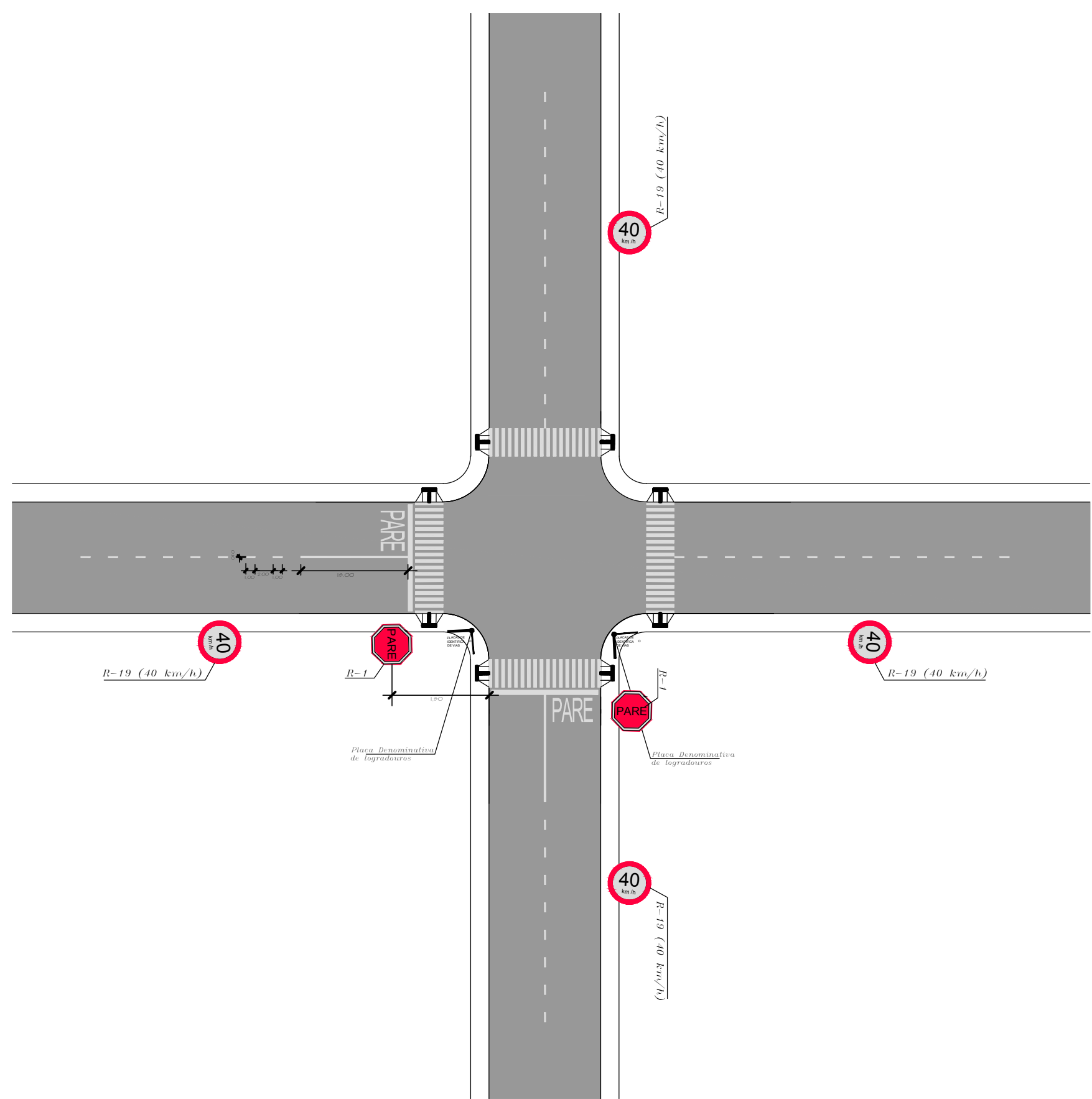
DETALHE SINALIZAÇÃO SEM ESCALA
