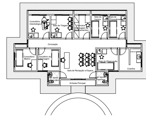
2 Planta Baixa UBS LAYOUT ESCALA 1:100
