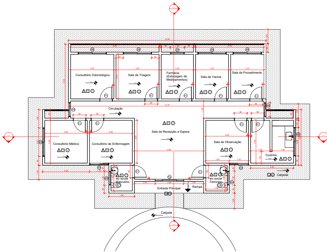
1 Planta Baixa UBS ESCALA 1:50
