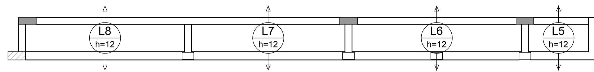
Armação positiva das lajes do pavimento TÉRREO (Eixo Y) escala 1:50
